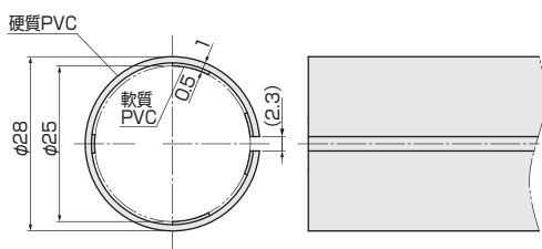
φ25パイプ装着時の製品寸法図
