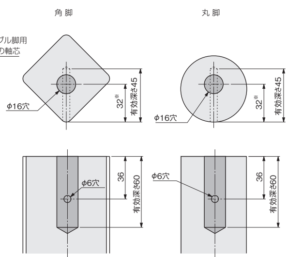
脚の加工寸法参考図
