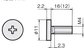
化粧ボルト
