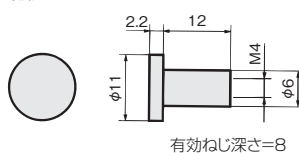
化粧ナット
