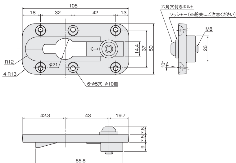
天板用金具
