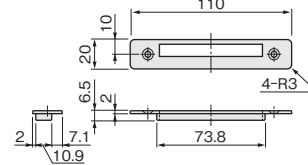
標準ガイド (サイズ20)
