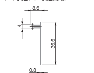
中間スクリーン (2本引違い、2枚連動用)
