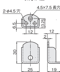
取付け座
