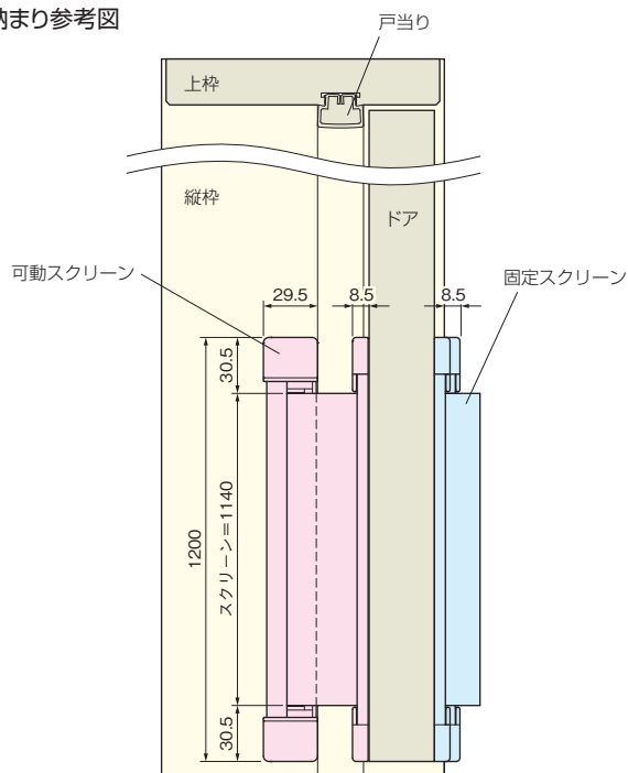
納まり参考図
