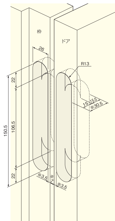
■ドアと枠の加工寸法参考図
