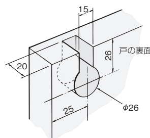
上り車の取付け加工寸法
