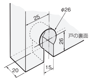
下り車の取付け加工寸法
