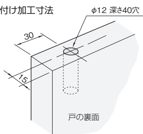
HD-14またはHD-16の取付け加工寸法
