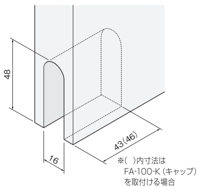
下部調整戸車の取付加工寸法
