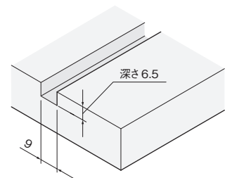
床/敷居の加工寸法
