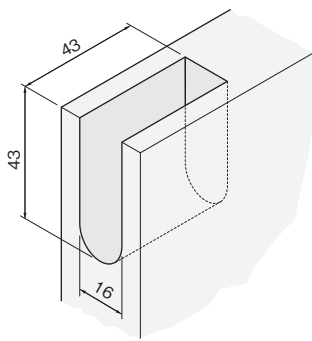
上部ガイドの取付け加工寸法
