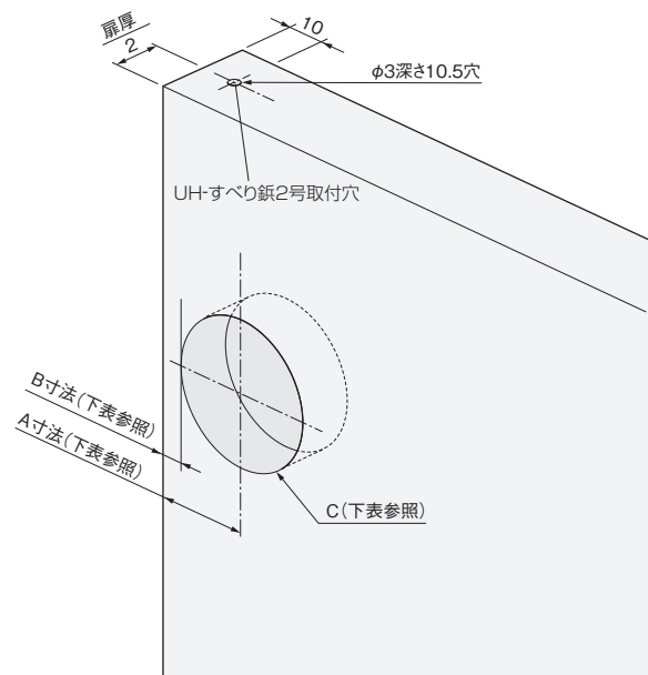
扉の加工、金具の取付寸法
