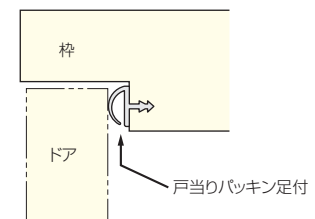
取付け図
