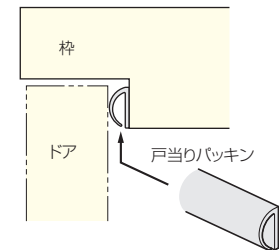
取付け図
