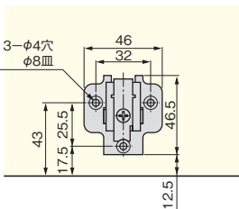
RBK-32座金
