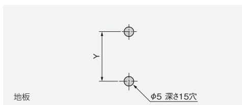
下部ガイドピン取付けのための「地板加工図」
