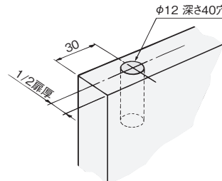
上下ピボットおよび案内ランナーの取付け加工寸法
