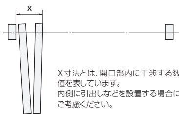
上下ピボットおよび案内ランナーの取付け加工寸法
