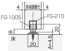
下部ガイド
