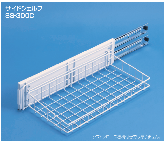
●写真・図面は左勝手仕様です。
