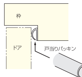
取付け図
