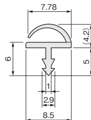
断面図
