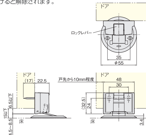
解除状態
