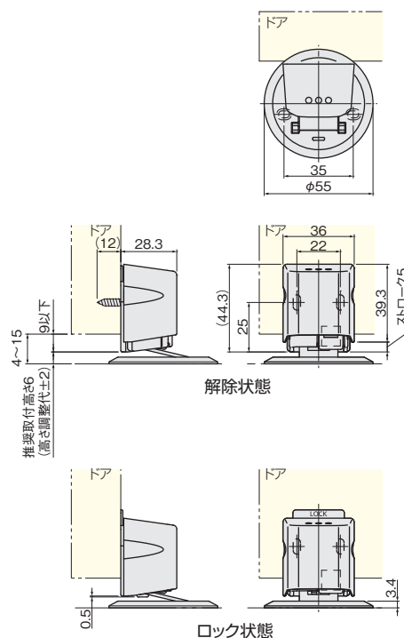
解除状態
