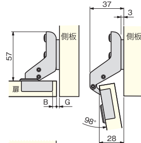
C105-0-6-CL インセットタイプ
