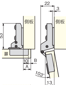
C105-14-6-CL 4-14 かぶせタイプ
