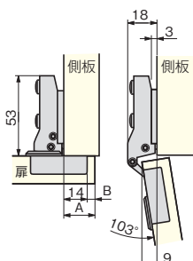
C105-18-6-CL 4-18 全かぶせタイプ
