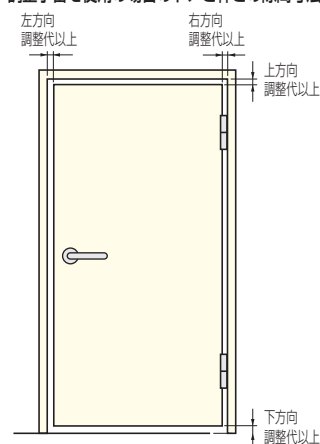
調整丁番を使用した場合のドアと枠との隙間寸法
