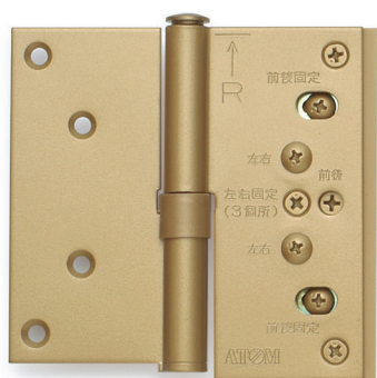
上用丁番。 左よりゴールド塗装、シルバー塗装、アンバー塗装
