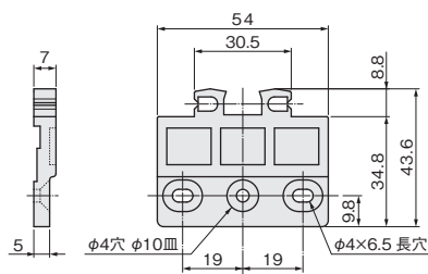
底付け受け (BL)
