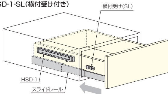
HSD-1-SL(横付け受け付き)
