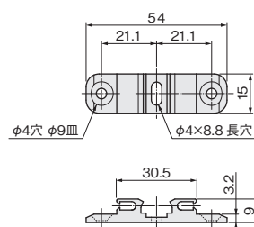
横付け受け (SL)
