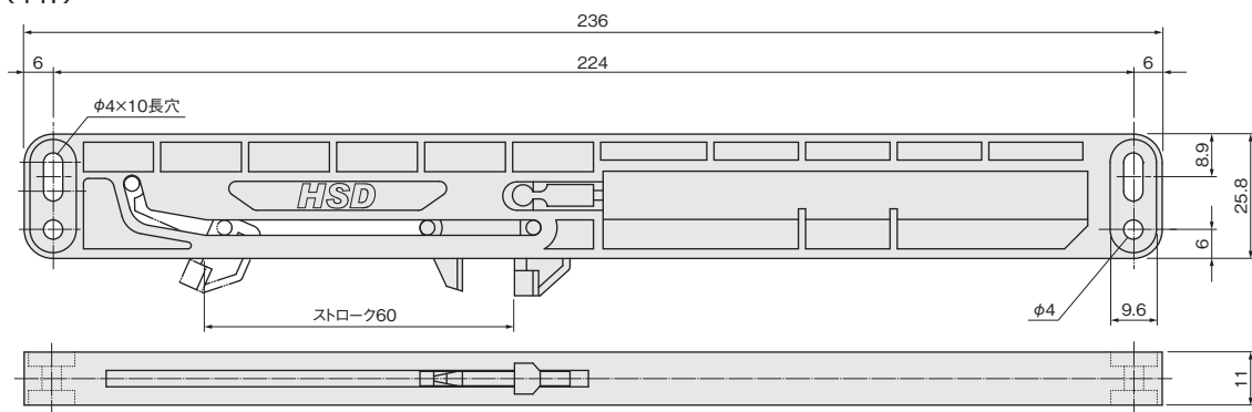
横付け受け (SL)
