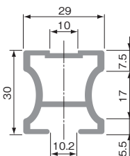
縦枠 30mm×29mm
