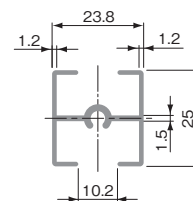
中棧
