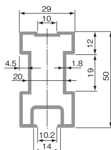
縦枠 50mm×29mm
