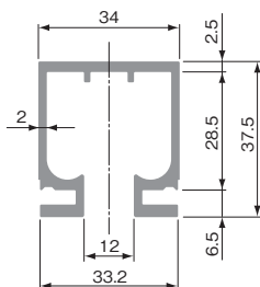
上部レール
