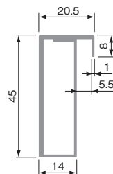
横枠
