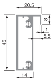
縦枠
