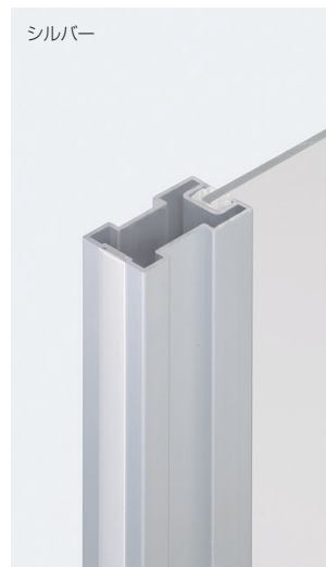
縦枠50mm×29mm
