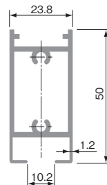
横枠(上、下)
