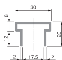
下部ガイドレール (2本引違い用)
