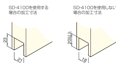
■戸の加工寸法参考図
