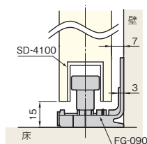
■金具の納まり参考図
