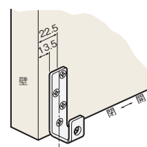
■金具の取付け位置
