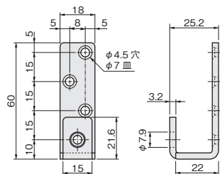
■金具の納まり参考図
