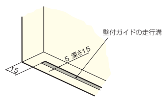
■戸下面の加工寸法参考図
