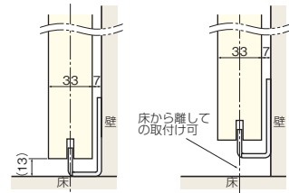
■金具の納まり参考図
