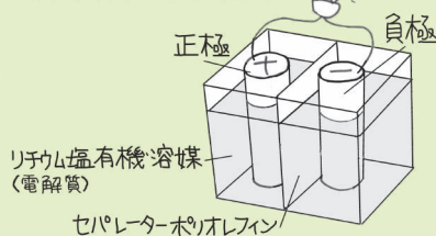
リチウムイオン電池の構造
