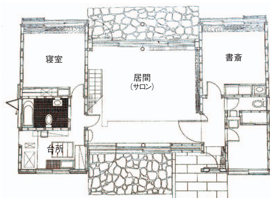
前川邸平面図
